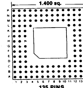
135 PINS Footprint 14011
