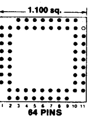
Footprint 11040
