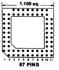
Footprint 11034
