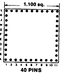
Footprint 11044
