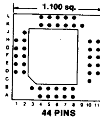
Footprint 11041
