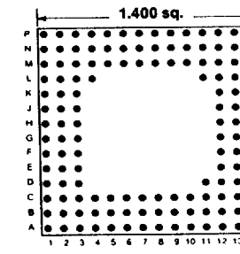
135 PINS Footprint 14012
