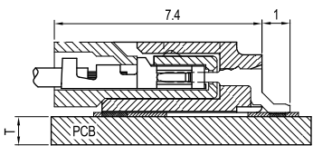
PCB ASS'Y
