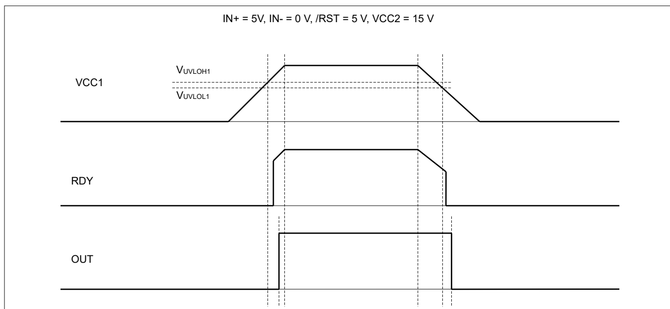
Figure 8 UVLO1
