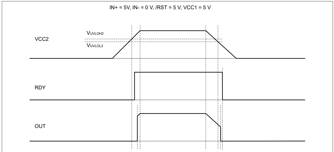
Figure 9 UVLO2
