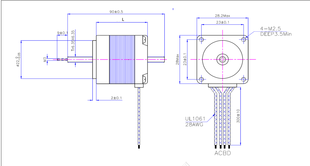
尺寸图 Mechanical Dimensions
