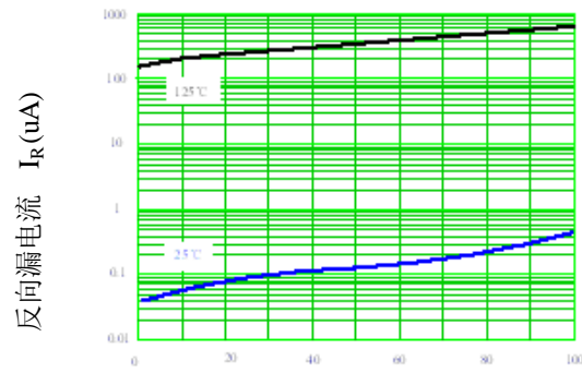
典型 I_R - V_R 关系特性(Per Diode)
