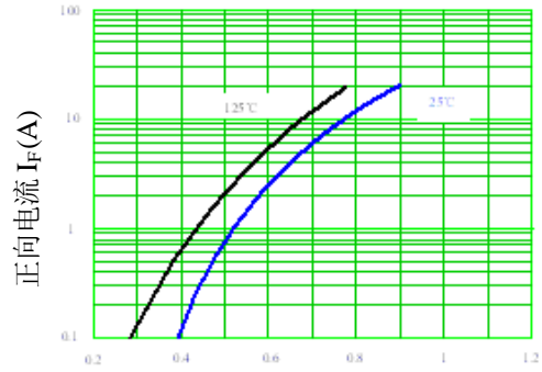
典型 I_F - V_F 关系曲线 (Per Diode)
