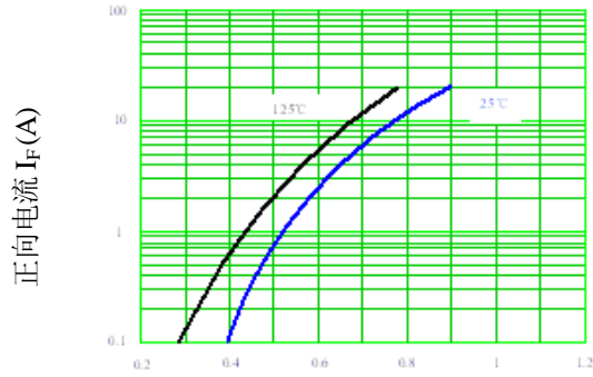
最大 I_F - V_F 关系曲线 (Per Diode)
