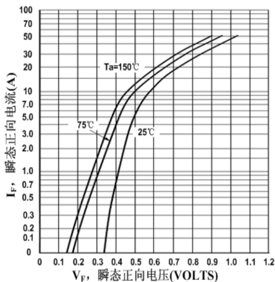
图(2) V_F - I_F 关系曲线 (Per Diode)
