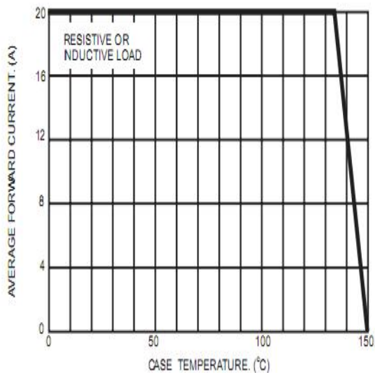
图(4) I_F - T_C 关系曲线 (Per Diode)
