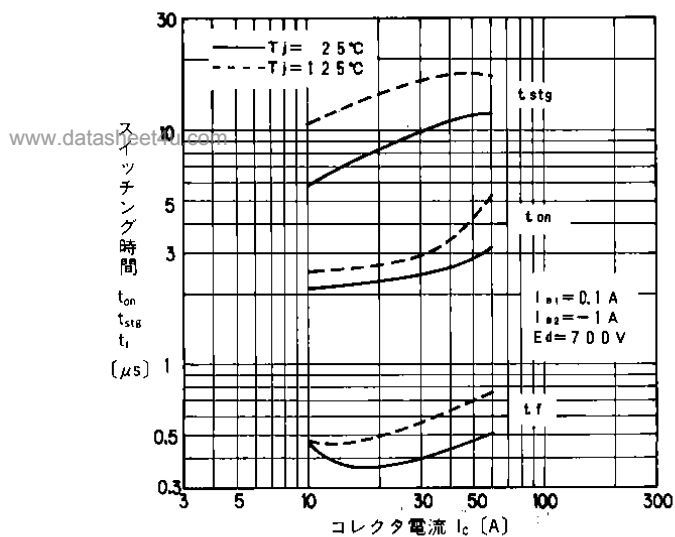
スイッチング時間—コレクタ電流特性 Switching Time
