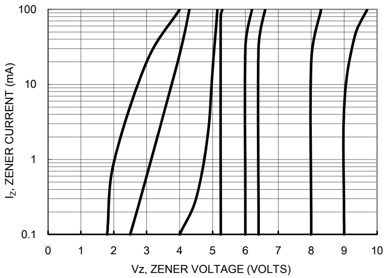
FIG. 6- V_z = 6.8 - 10 VOLTS
