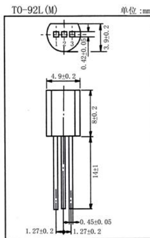
引脚: 1. E 2. C 3. B
