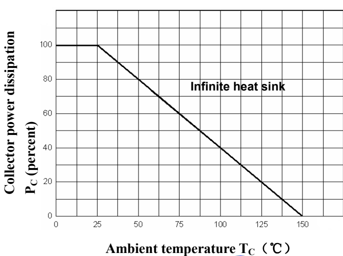
P_C - T_C
