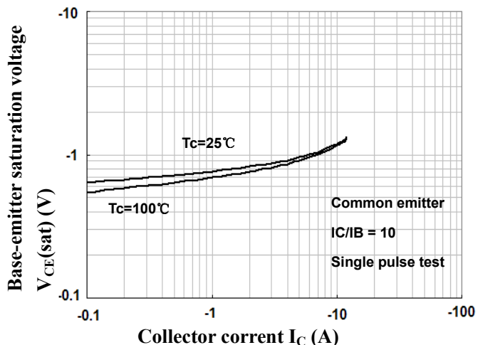
V_{BE(sat)} - I_C
