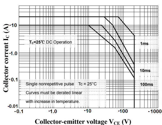
SOA
