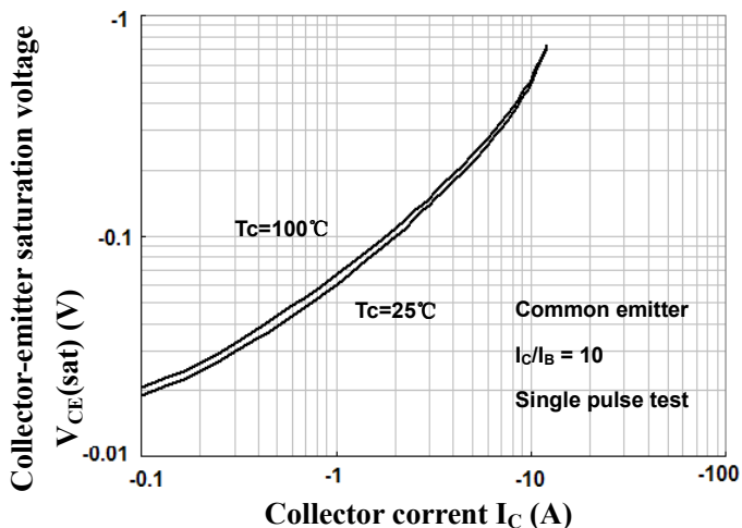
V_{CE(sat)} - I_C
