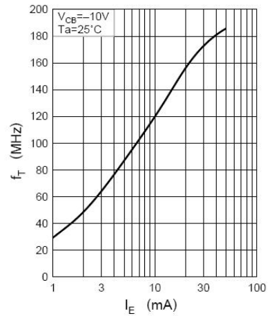
f_T - I_E
