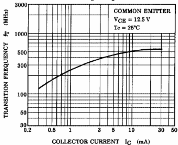
f_T - I_C
