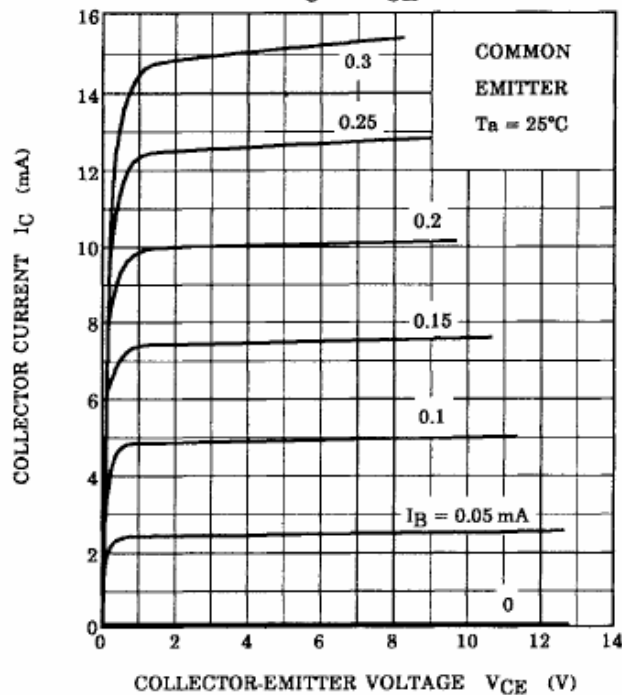
I_C - V_{CE}
