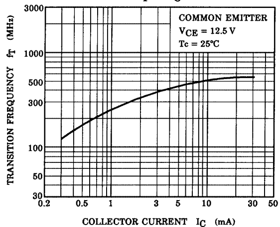
f_T - I_C
