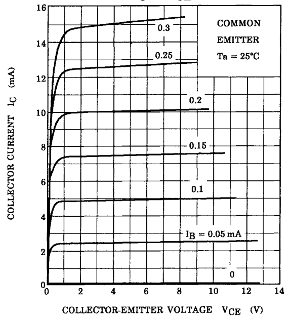
I_C - V_{CE}
