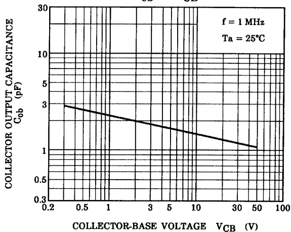
C_{ob} - V_{CB}
