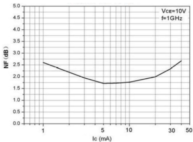
Fig 5. NF vs. I_c
