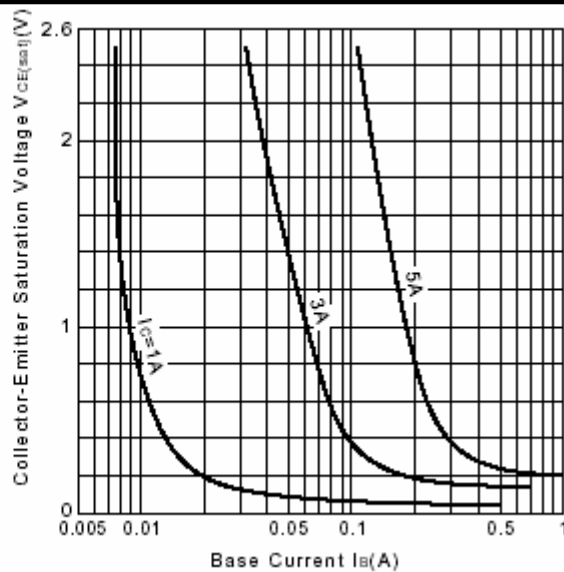
Fig.4 V_{CE(sat)}-I_B
