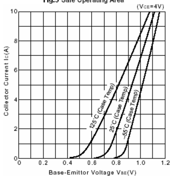
Fig.7 I_C - V_{BE}
