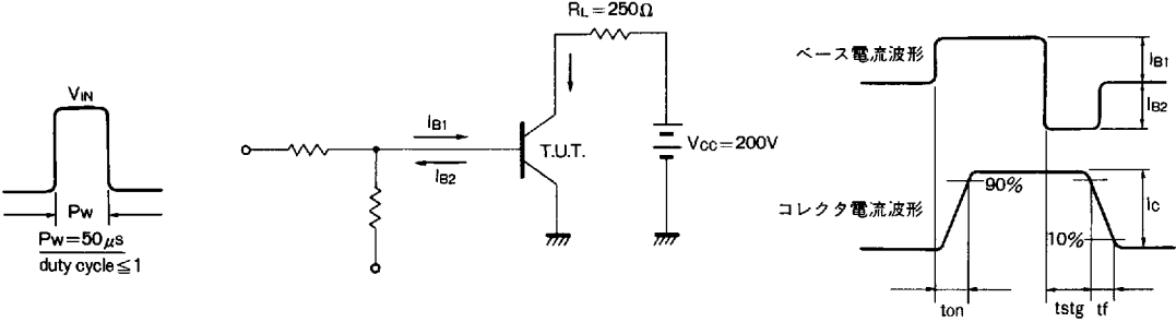
スイッチング時間測定回路図
