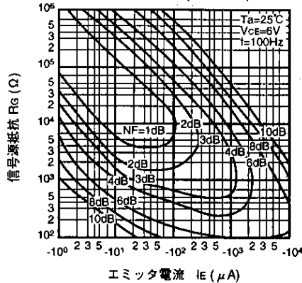
雑音指数特性 ( f=100\text{Hz} )
