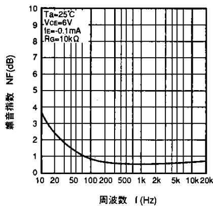
雑音指数一周波数特性
