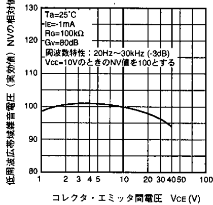
低周波広帯域雑音電圧 (実効値) — コレクタ・エミッタ間電圧特性
