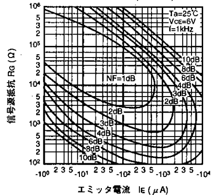
雑音指数特性 ( f=1\text{kHz} )
