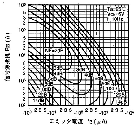
雑音指数特性 ( f=10\text{Hz} )
