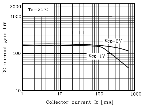
Fig. 5 h_{FE} - I_c
