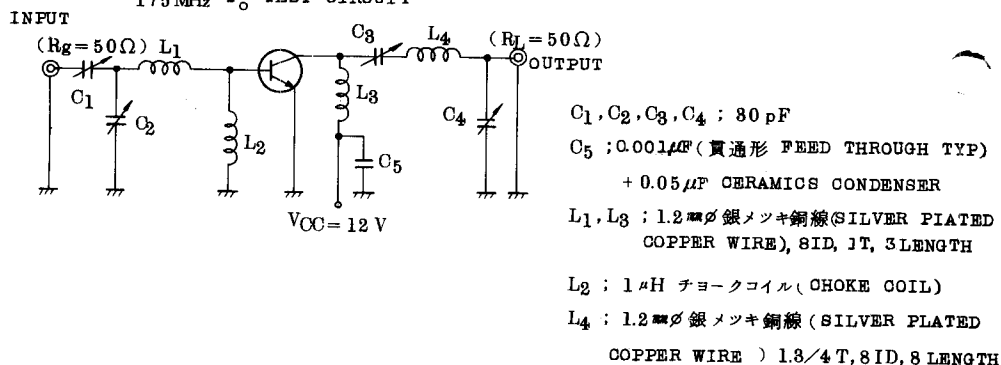
(Fig. 1) 175MHz 出力電力測定回路
