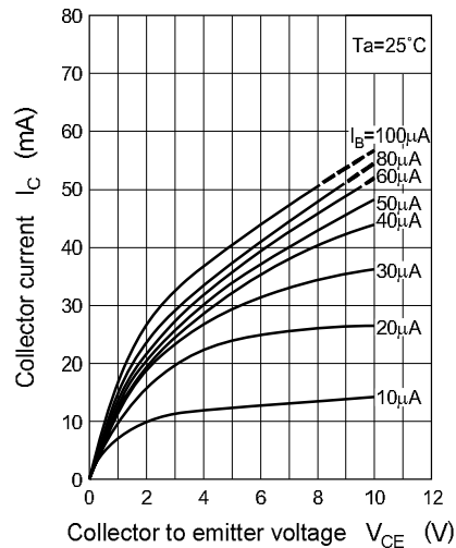
I_C - V_{CE}
