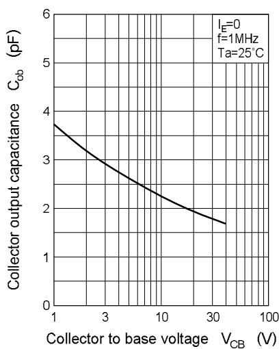
C_{ob} - V_{CB}
