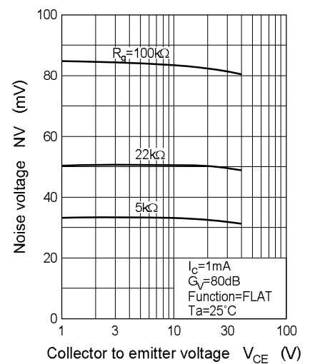
NV - V_{CE}
