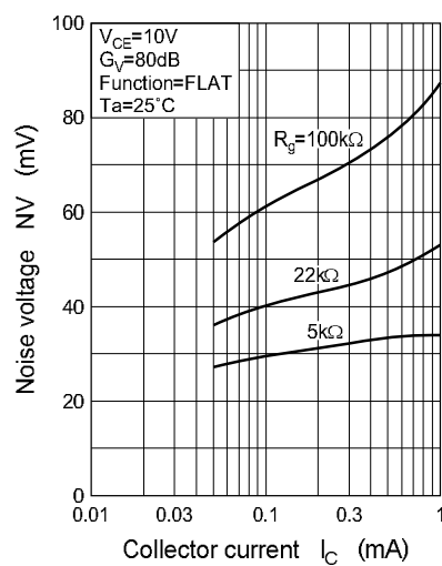
NV - I_C
