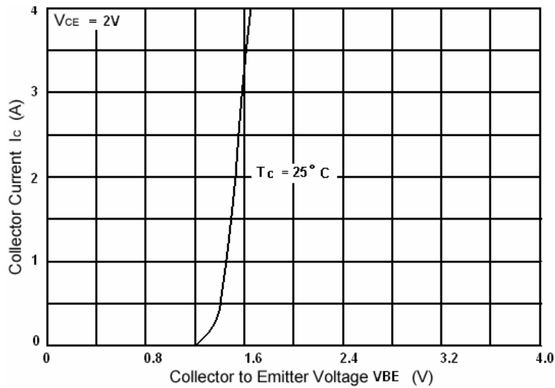
Fig.7 I_C - V_{BE}
