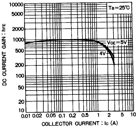
Fig.5 直交流増幅率-コレクタ電流特性
