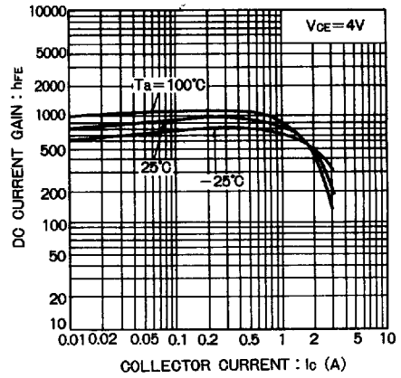
Fig.6 直交流増幅率-コレクタ電流特性
