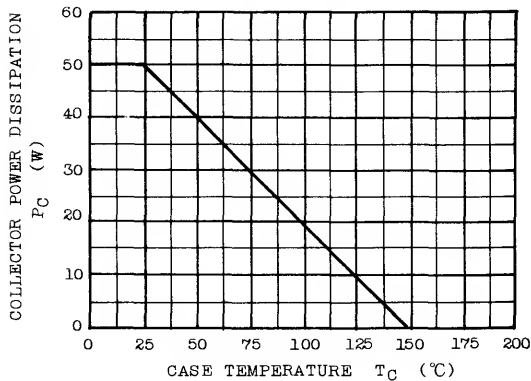
P_C - T_C
