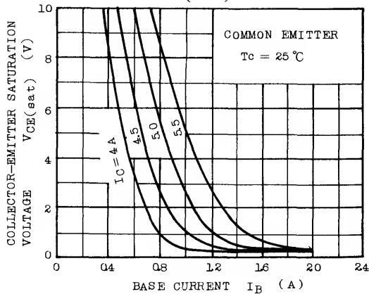
V_{CE(sat)} - I_B
