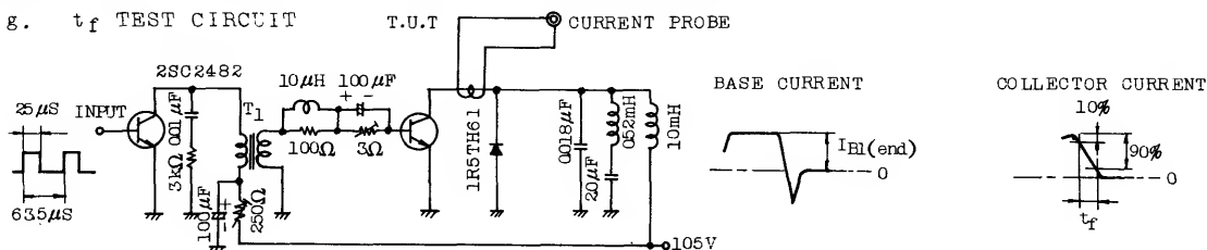
Fig. t_f TEST CIRCUIT
