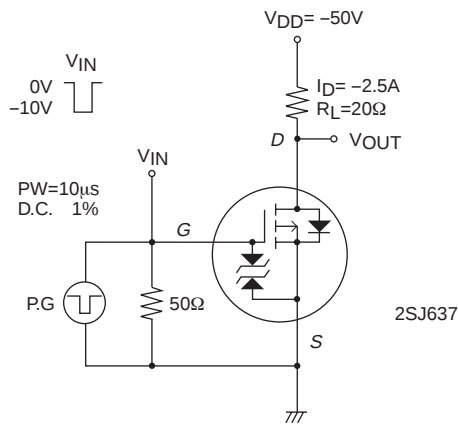
スイッチングタイム測定回路図
