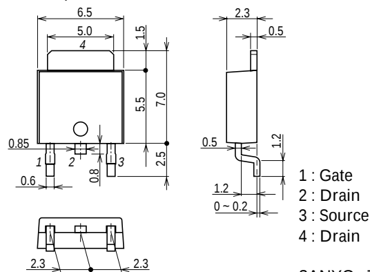
外形図 2092B
