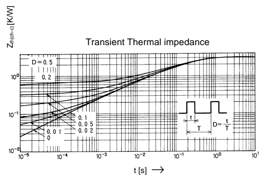
Zth(jc-0)
