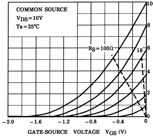
I D - V GS
