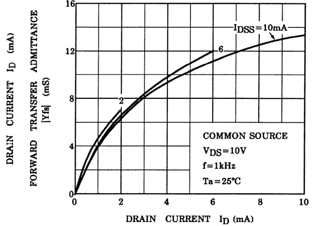
|Y fs | - I D
