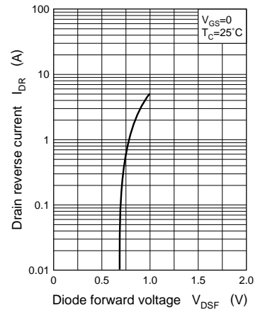
I_{DR} - V_{DSF}
