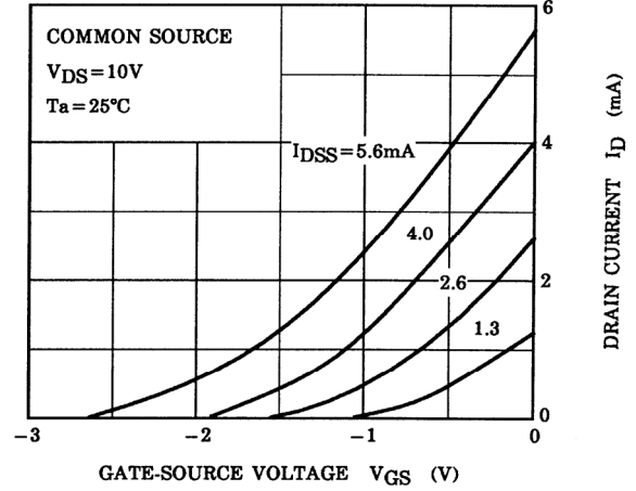
I_D - V_{GS}
