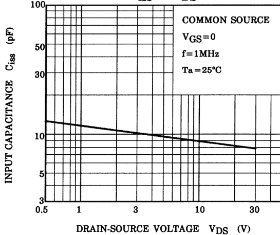
C_{iss} - V_{DS}
