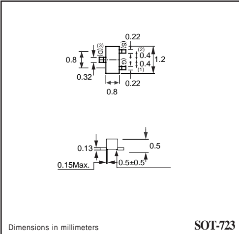
SOT-723
