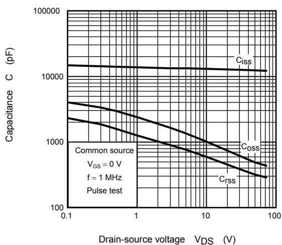
Capacitance - V_{DS}
