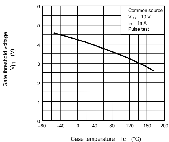
V_{th} - T_c
