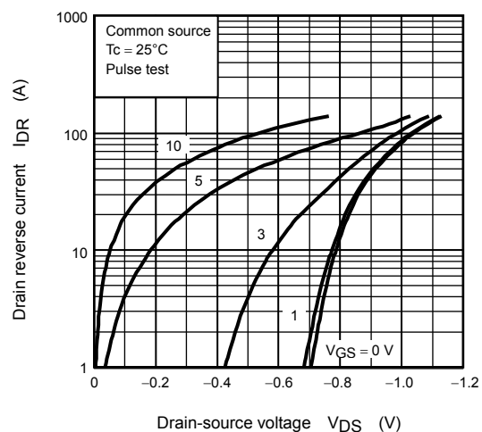
I_{DR} - V_{DS}
