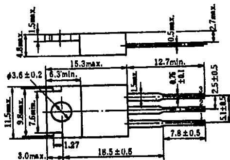
(JEDEC TO-220AB)
