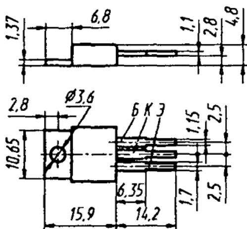
2Т819(А2-В2), КТ819(А-Г)
