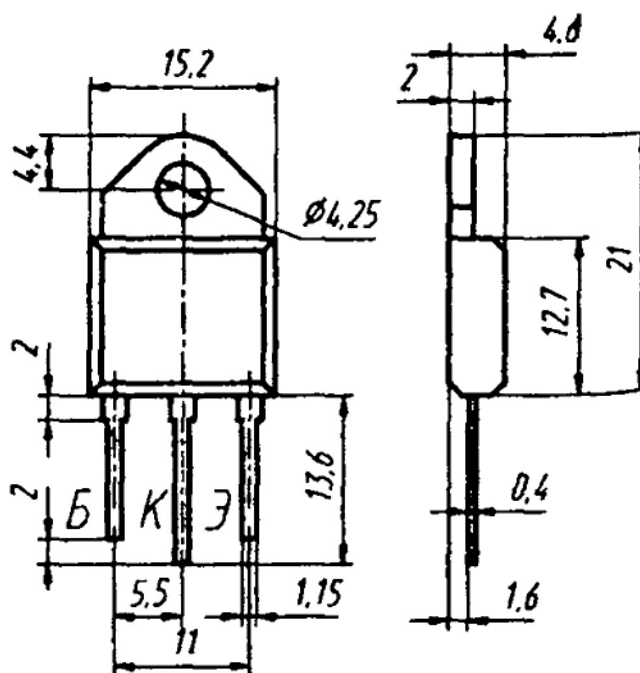
КТ819(А1-Г1)
