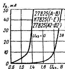
Входные характеристики
