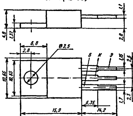
2Т825 (А2-В2)
