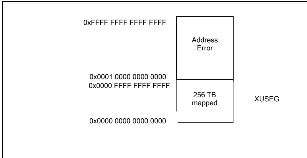
图 5-3 用户模式下用户虚拟地址空间概况
