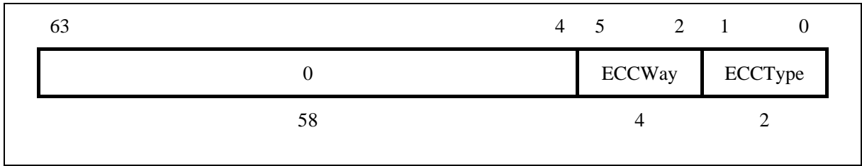
图 3-32 CacheErr 寄存器
