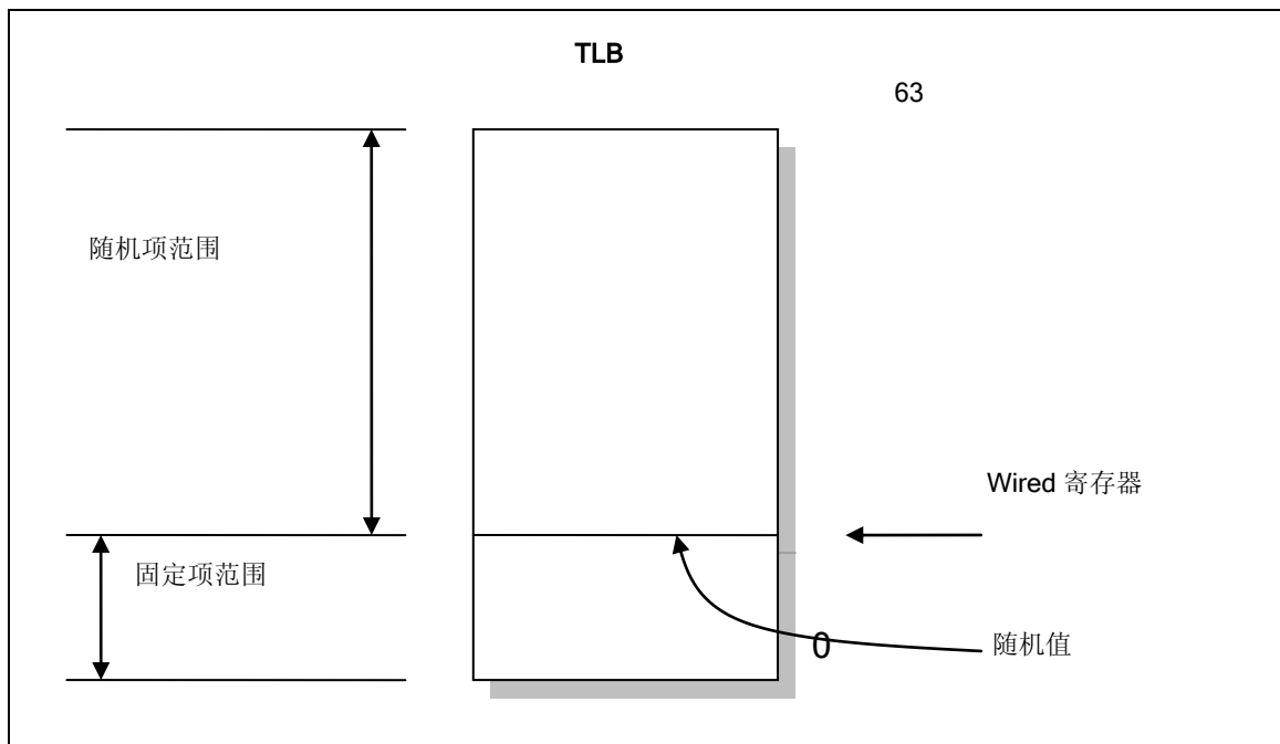
图 3-7 Wired 寄存器界限
