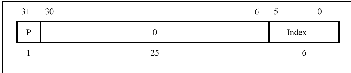
图 3-1 Index 寄存器
