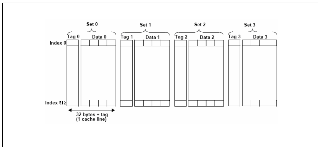
图 4-3 数据 Cache 的组织结构
