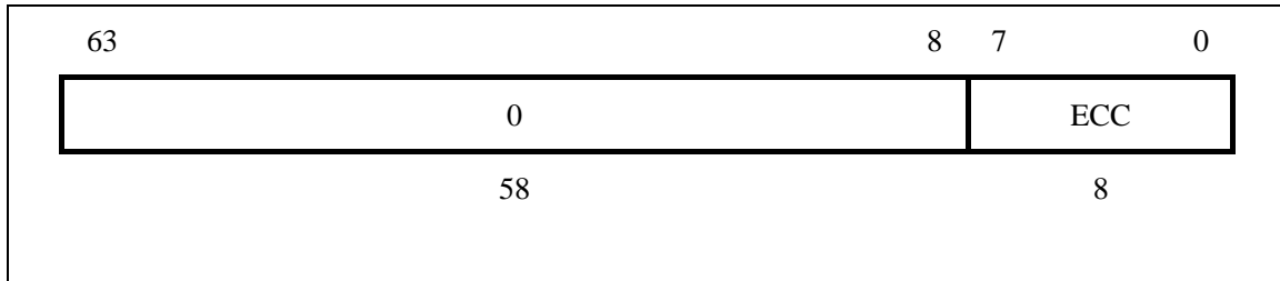
图 3-31 ECC 寄存器
