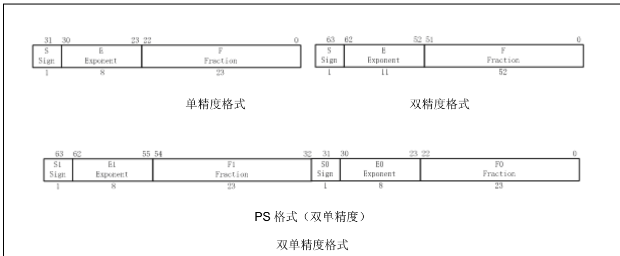
图 7-8 浮点格式
