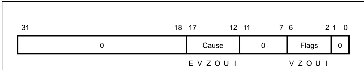
图 7-6 FEXR 寄存器
