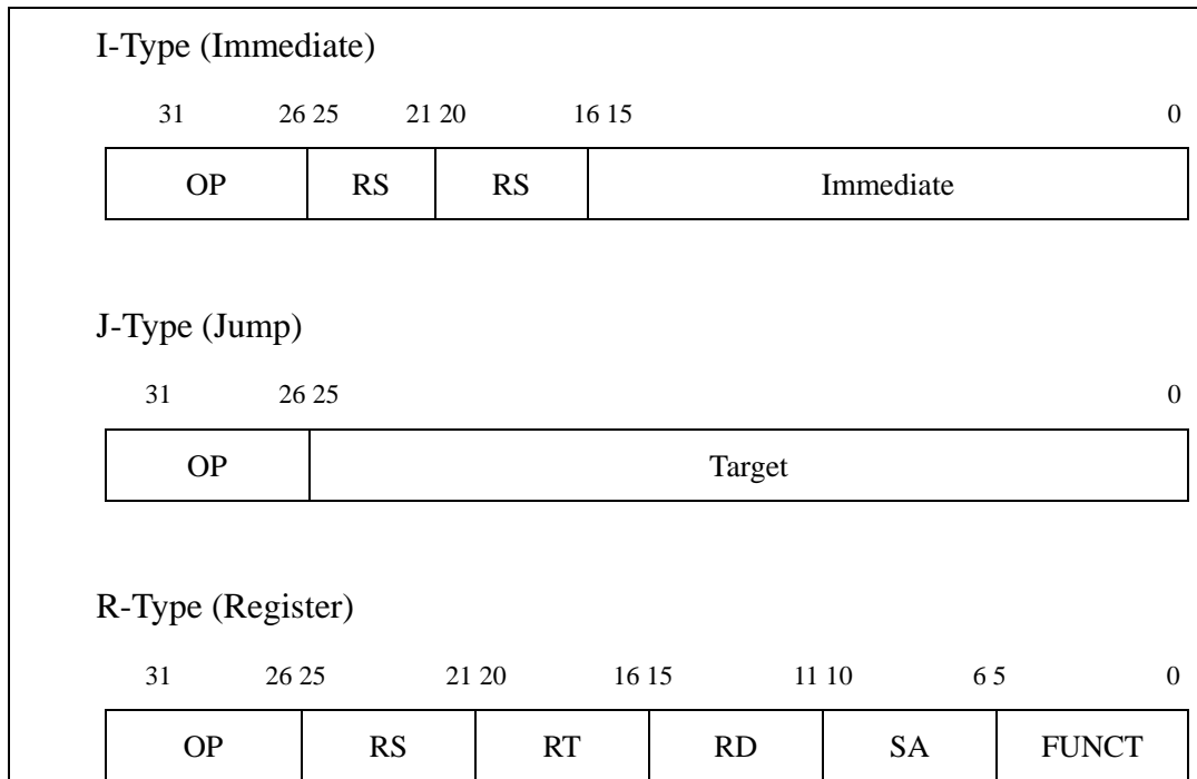
图 2-1 CPU 指令格式
