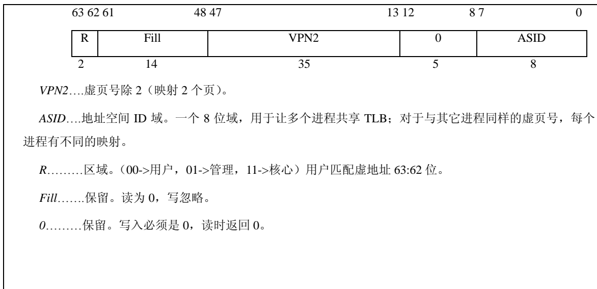
图 5-8 EntryHi 寄存器
