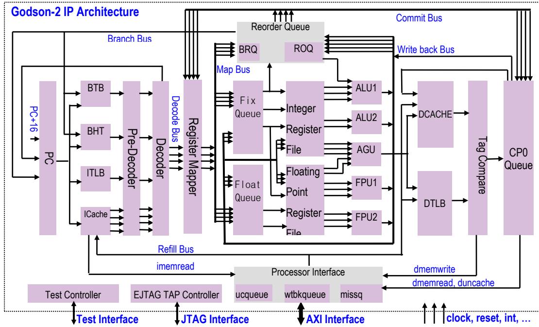
图 1-1 GS464 处理器的基本结构
