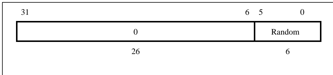
图 3-2 Random 寄存器
