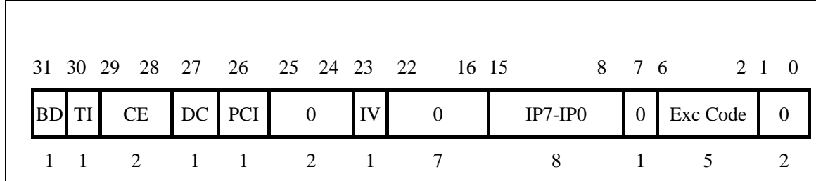
图 3-17 Cause 寄存器
