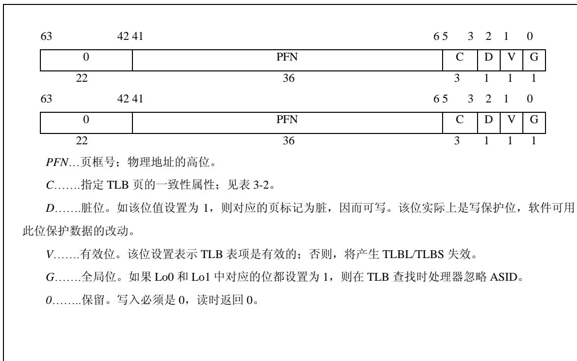
图 5-9 EntryLo0 和 EntryLo1 寄存器
