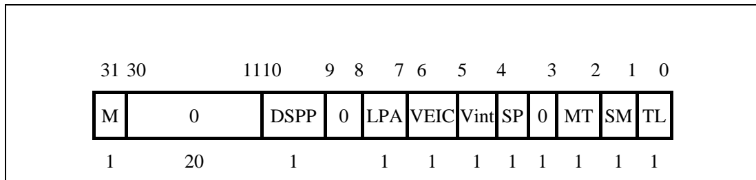
图 3-24 Config3 寄存器
