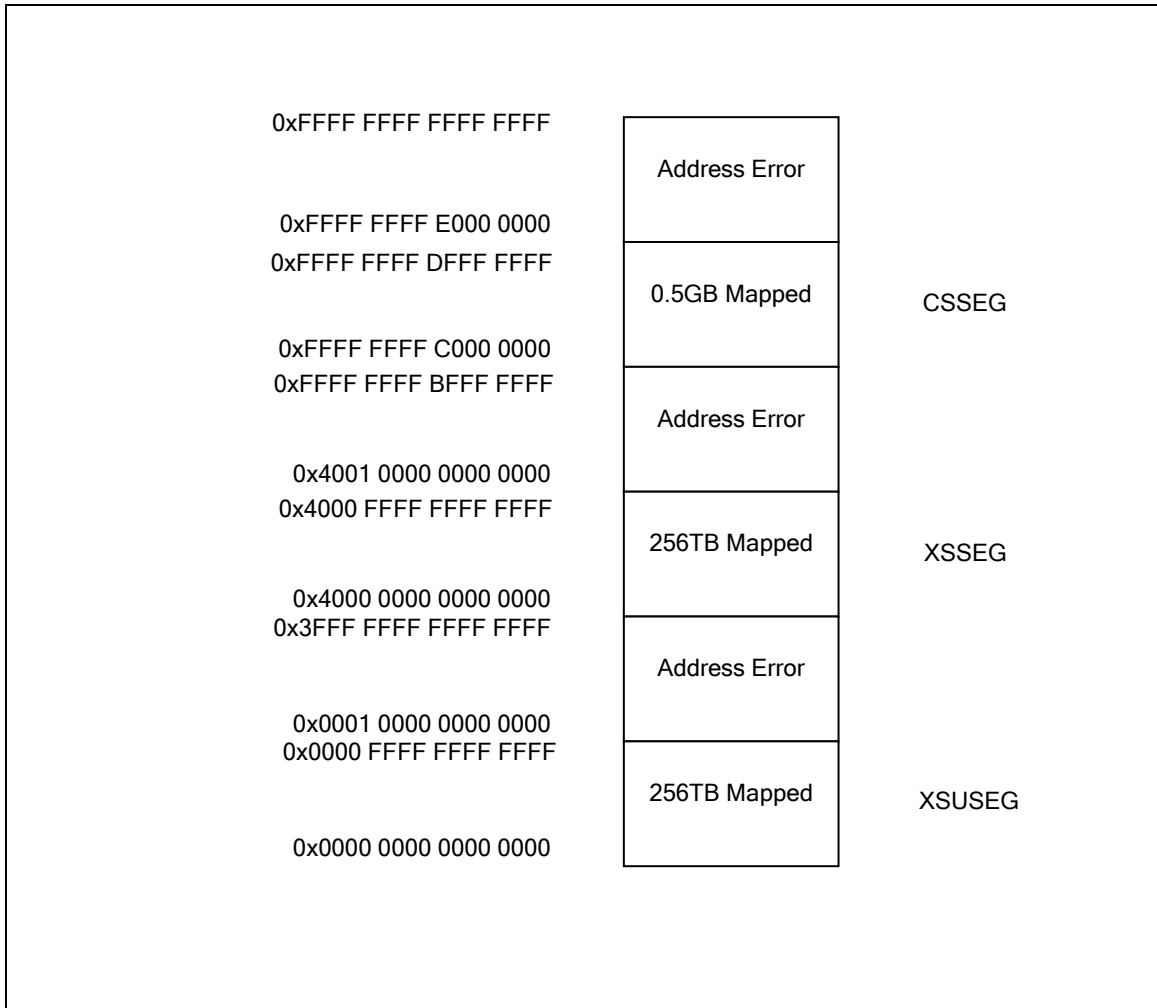
图 5-4 管理模式下用户空间和管理空间
