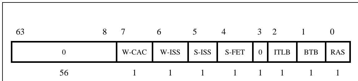
图 3-27 Diagnostic 寄存器
