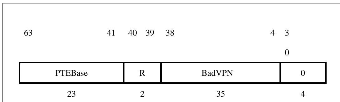
图 3-26 XContext 寄存器
