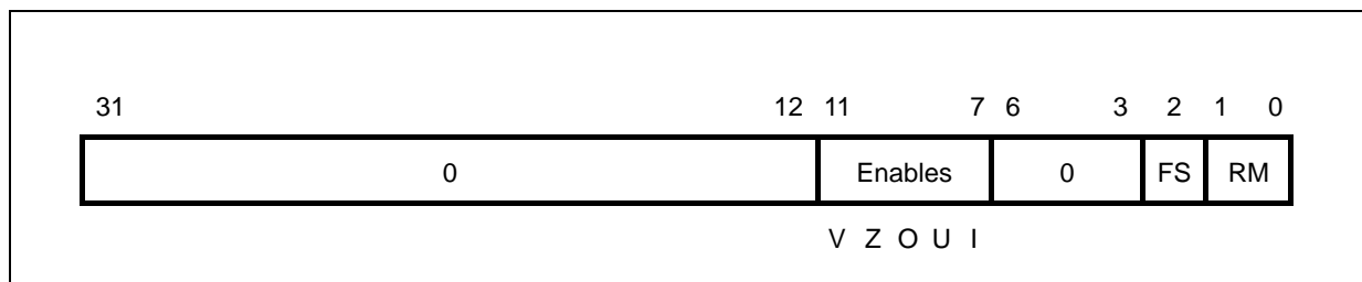
图 7-7 FENR 寄存器
