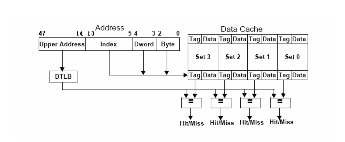
图 4-4 数据 Cache 访问
