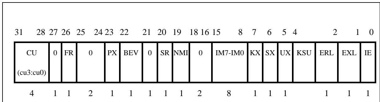
图 3-14 Status 寄存器
