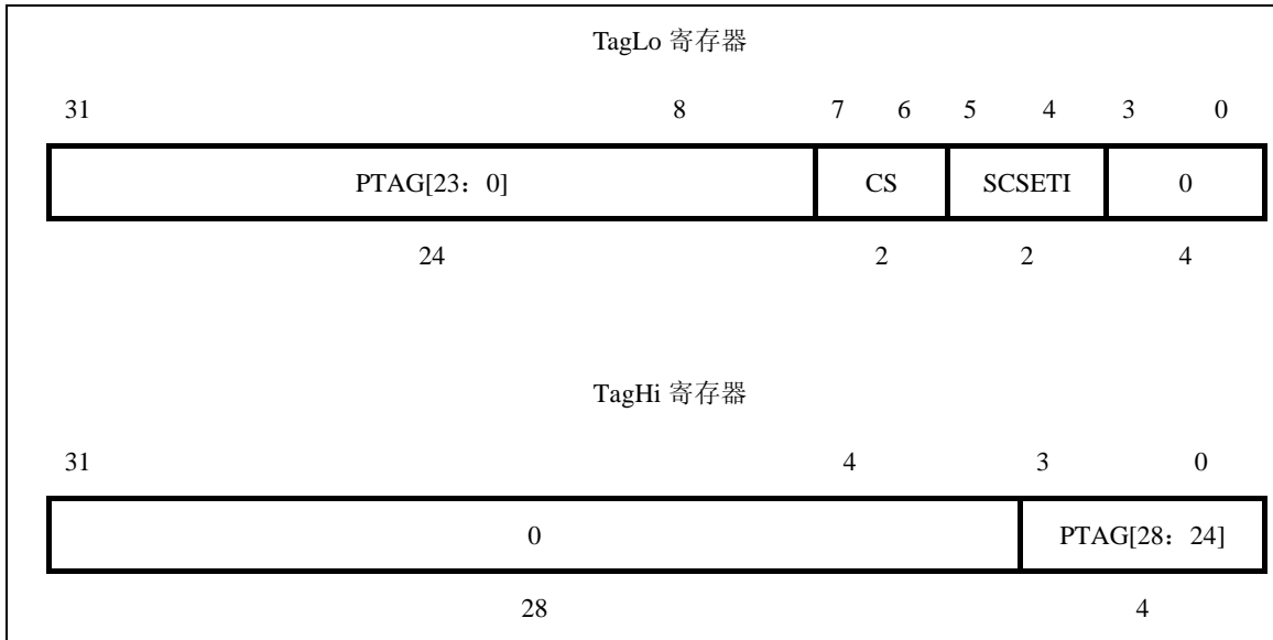
图 3-34 TagLo 和 TagHi 寄存器(P-Cache)
