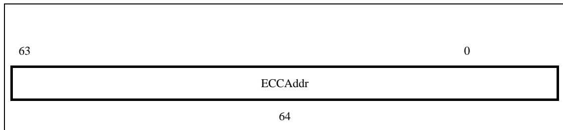
图 3-33 CacheErr1 寄存器
