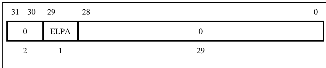
图 3-6 PageGrain 寄存器
