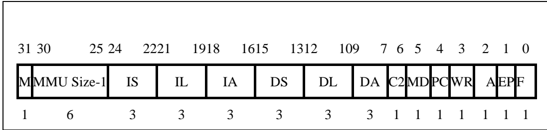
图 3-22 Config1 寄存器
