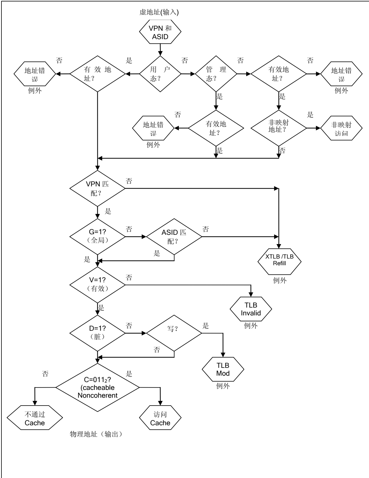
图 5-10 TLB 地址转换
