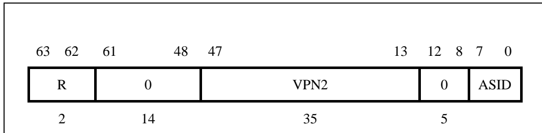
图 3-13 EntryHi 寄存器
