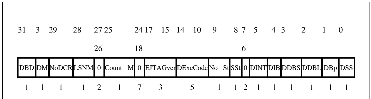
图 3-28 Debug 寄存器
