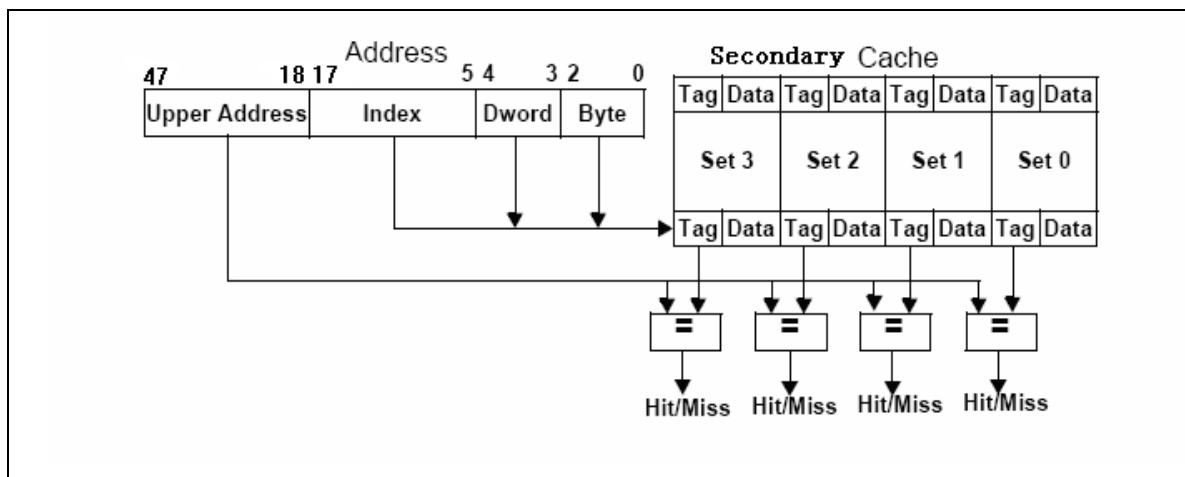
图 4-5 二级 Cache 访问
