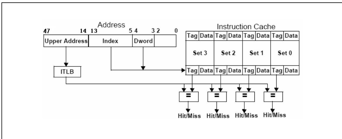
图 4-2 指令 Cache 访问
