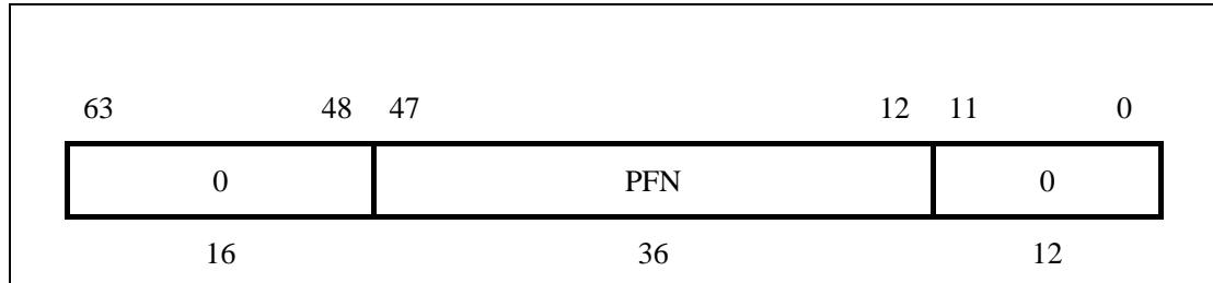
图 3-25 LLAddr 寄存器
