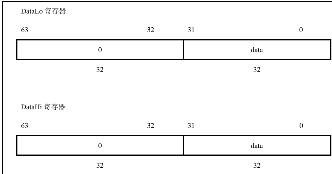
图 3-35 DataLo 和 DataHi 寄存器
