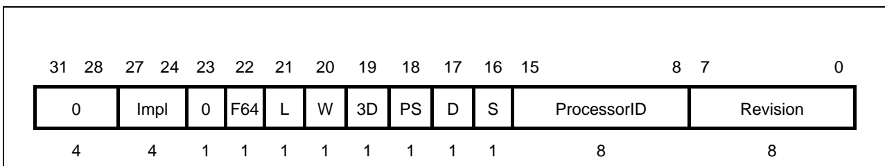
图 7-3 FIR 寄存器
