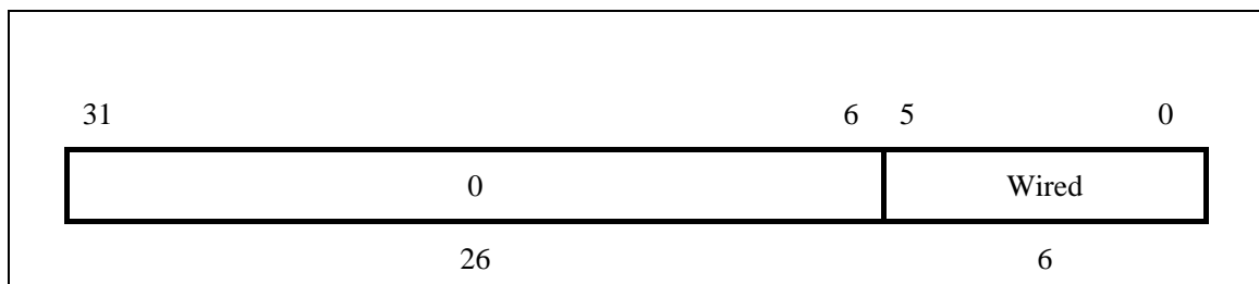
图 3-8 Wired 寄存器
