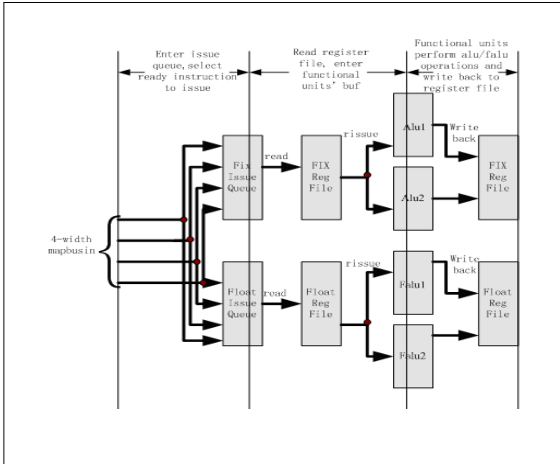
图 7-1 龙芯 3A1000 体系结构中功能单元的组织构成
