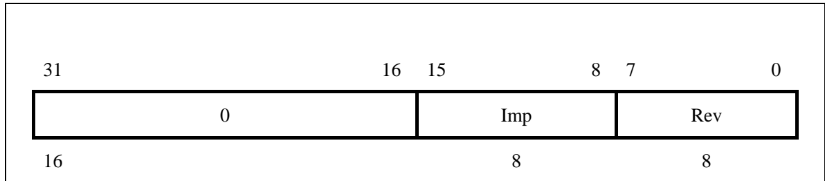
图 3-19 Processor Revision Identifier 寄存器
