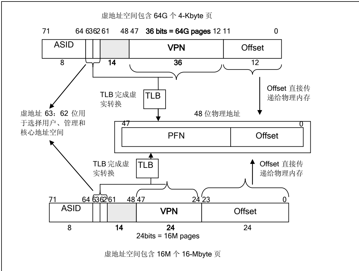
图 5-2 64 位模式虚拟地址转换
