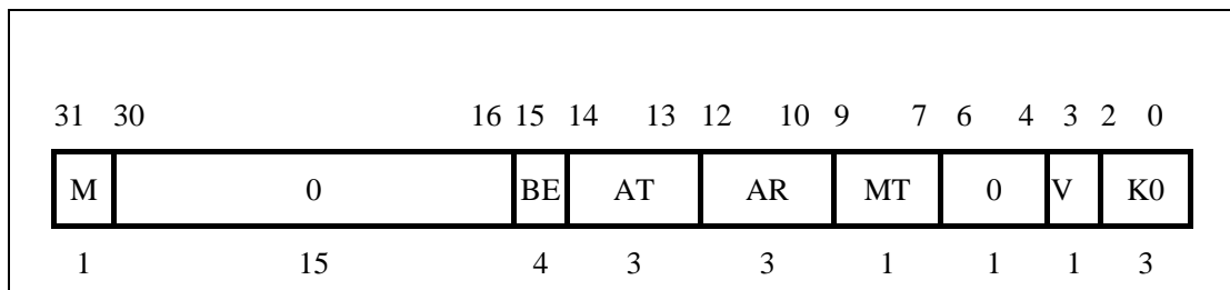
图 3-21 Config 寄存器
