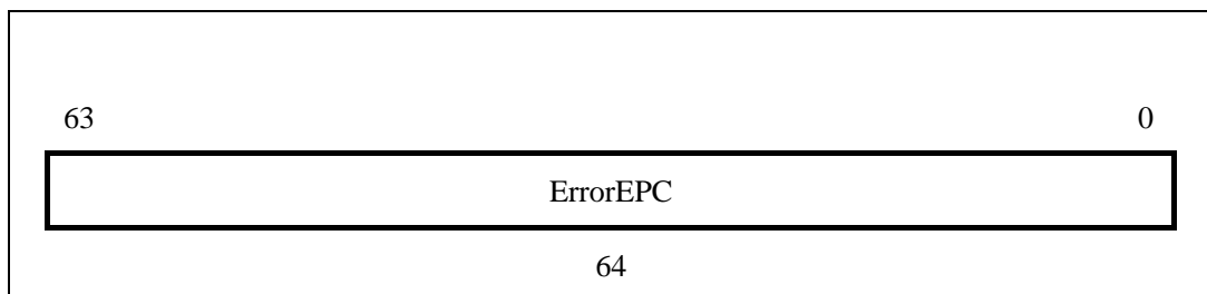
图 3-36 ErrorEPC 寄存器
