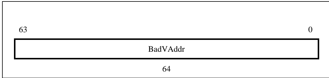
图 3-10 BadVAddr 寄存器
