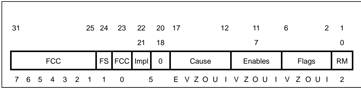
图 7-4 FCSR 寄存器
