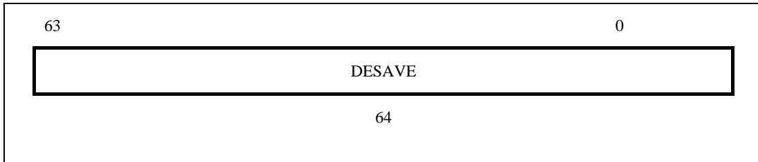
图 3-37 DESAVE 寄存器
