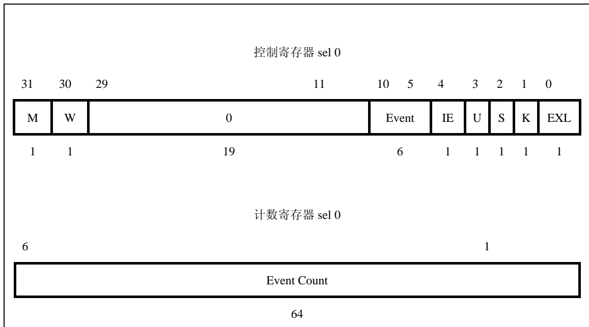
图 3-30 性能计数器寄存器
