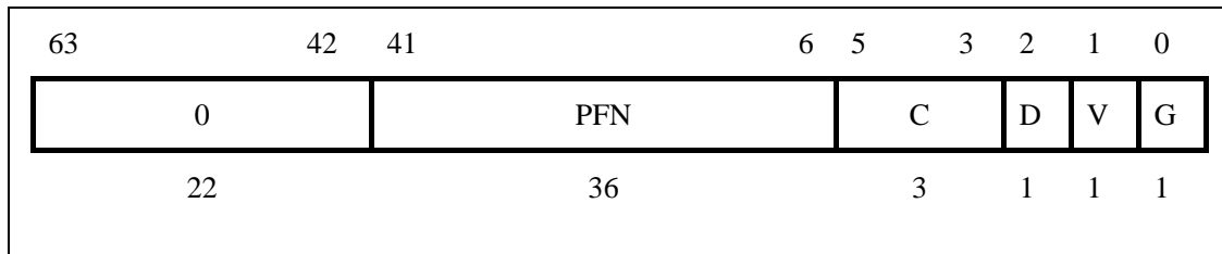
图 3-3 EntryLo0 和 EntryLo1 寄存器
