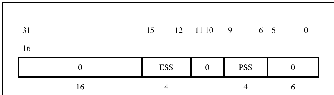
图 3-16 SRSCtl 寄存器
