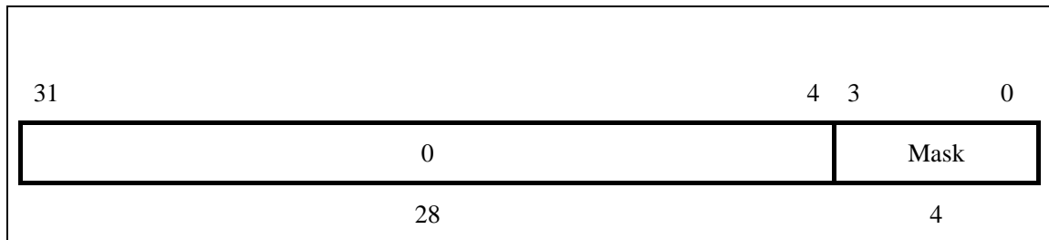
图 3-9 HWREna 寄存器
