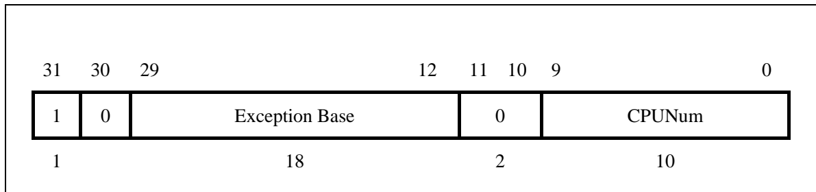
图 3-20 Ebase 寄存器
