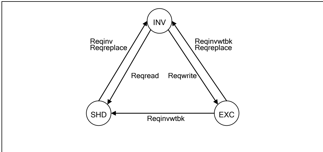
图 4-6 龙芯 3 号 cache 状态转换
