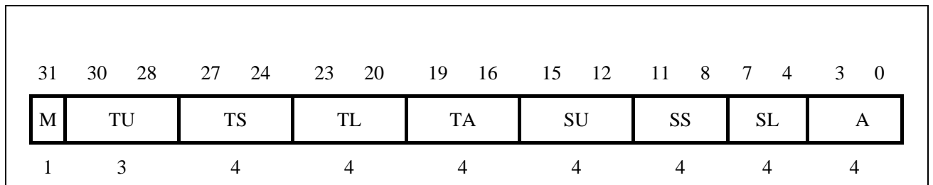
图 3-23 Config2 寄存器
