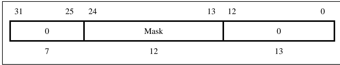
图 3-5 PageMask 寄存器
