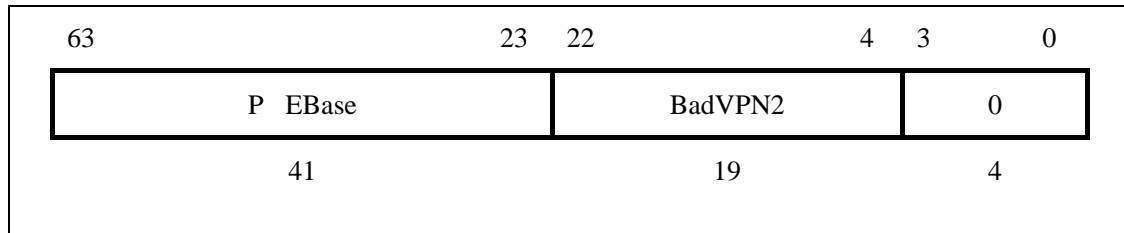
图 3-4 Context 寄存器
