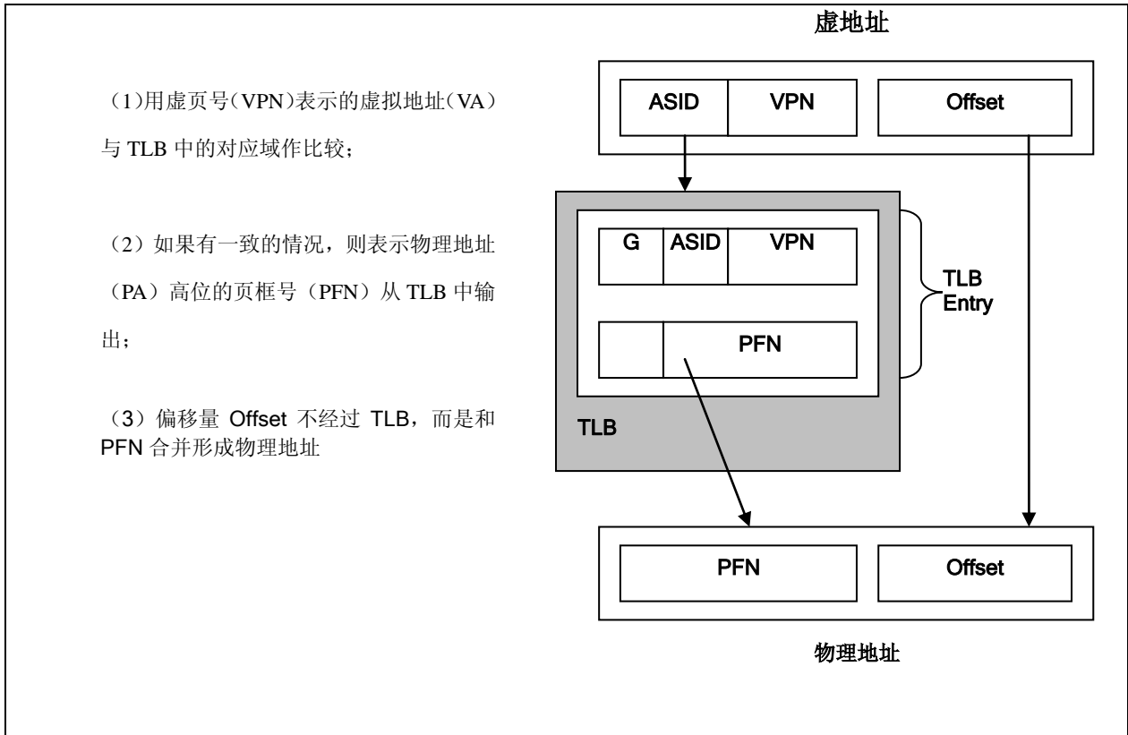
图 5-1 虚实地址转换概览
