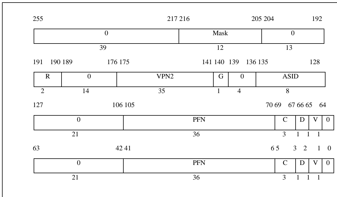
图 5-6 TLB 表项
