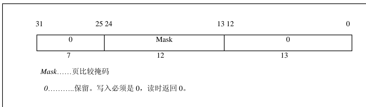
图 5-7 PageMask 寄存器
