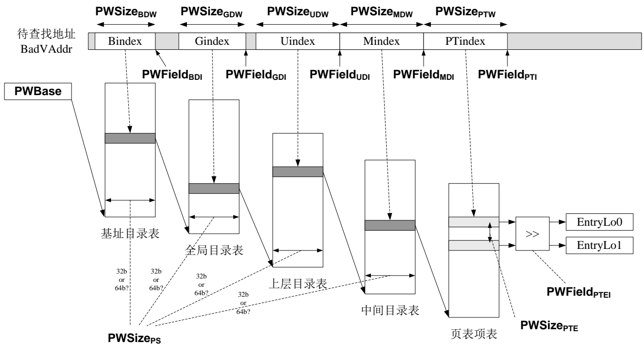
图 7-9 PWBase, PWField, PWSize 与 PWCtl 所支持的页表访问过程
