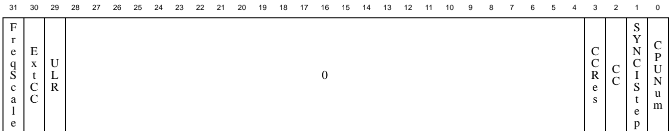
图 7-16 HWREna 寄存器格式
