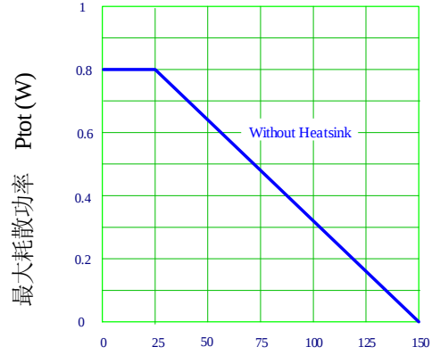
环境温度 T_a ( ^\circ\text{C} )
