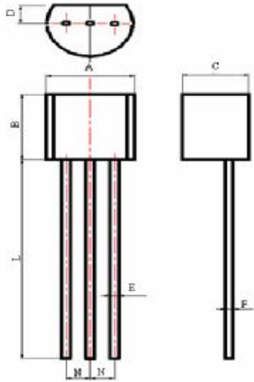
外形图: TO-92
