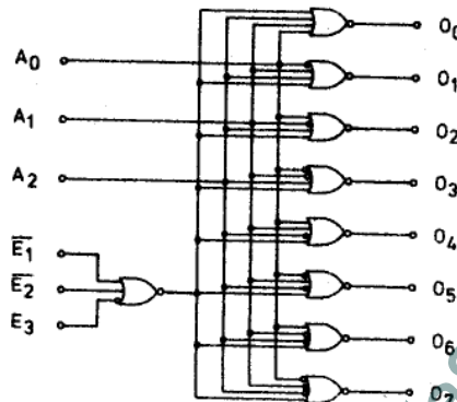
Schemat logiczny
