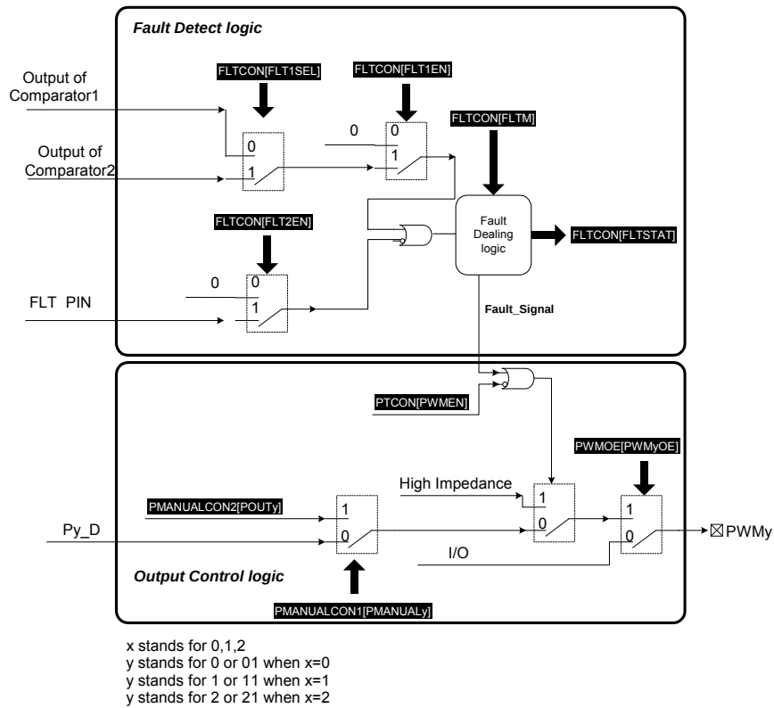
图8-1-14 输出控制与故障检测逻辑简图
