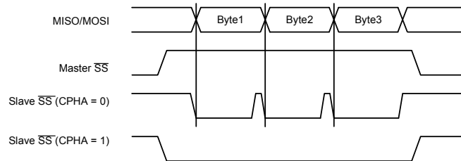
CPHA/SS时序
