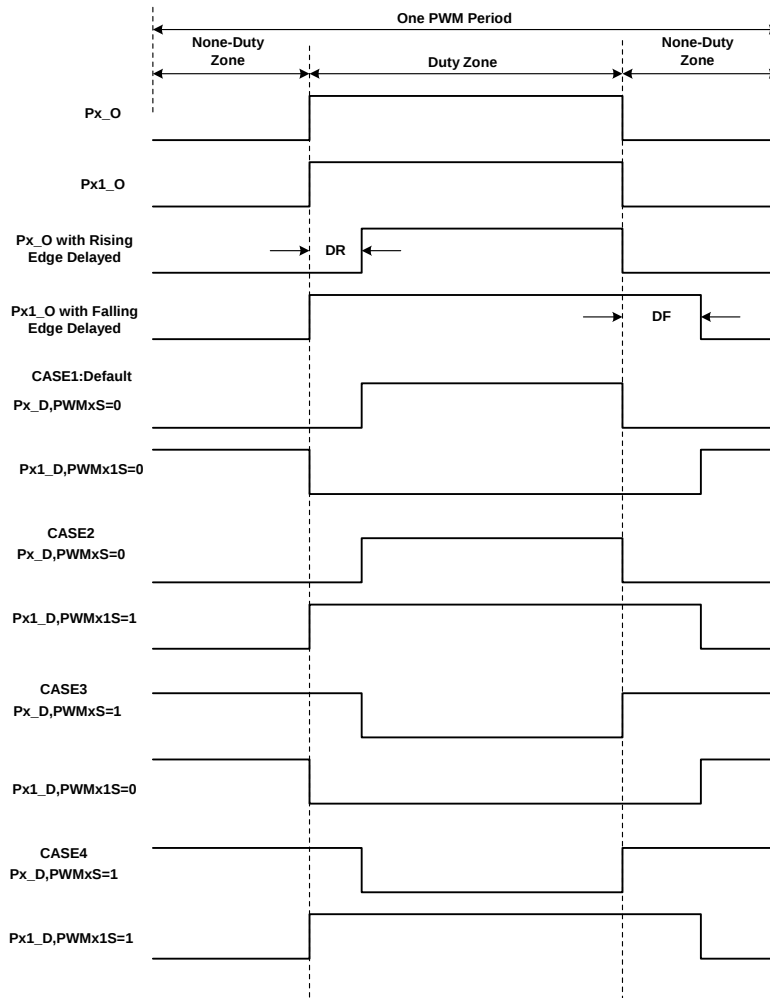
图8-1-13 不同极性设置下的死区波形
