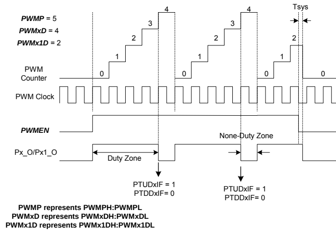
图8-1-7 边沿对齐计数、互补输出模式下的PWM原始波形
