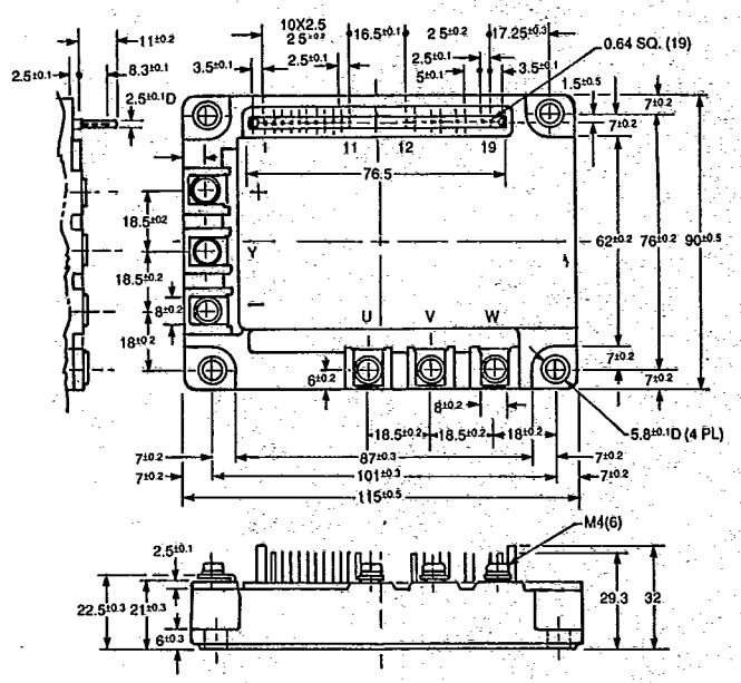
PKG.2
