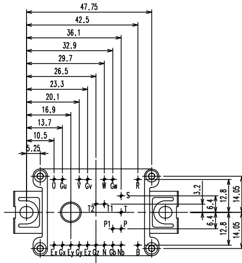
断面 A-A (1.5 : 1) SECTION A-A
