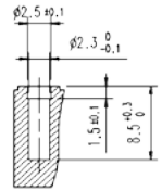
断面 A-A (1.5 : 1) SECTION A-A
