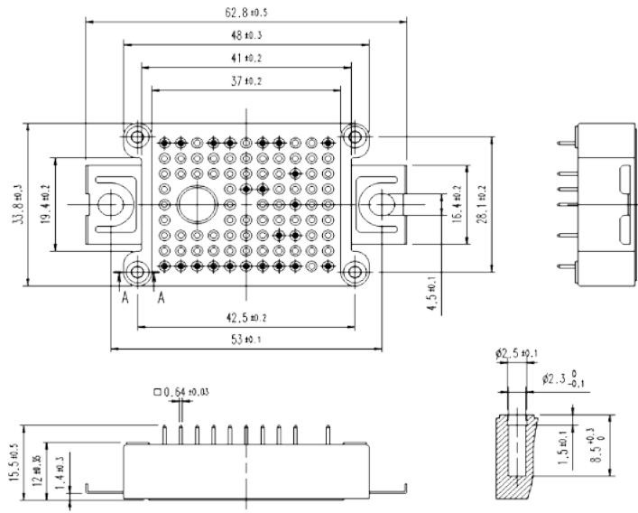
断面 A-A (1.5 : 1) SECTION A-A
