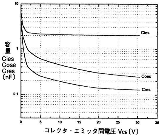
容量-コレクタ・エミッタ間電圧特性(Tj=25°C)〈ブレーキ部〉 Capacitance vs. Collector-Emitter voltage<BRAKE>
