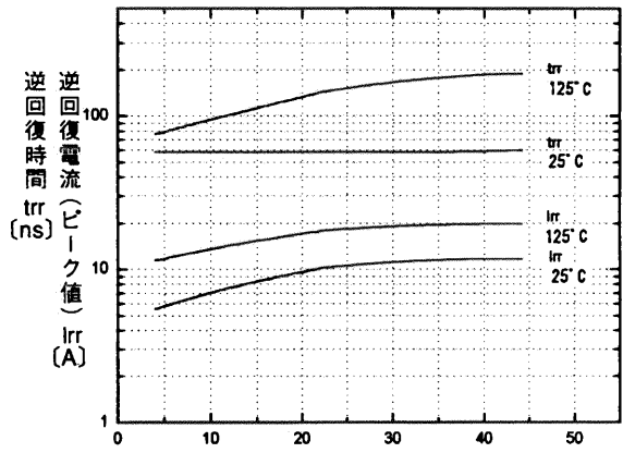
順電流 I_F [A] T_{rr} , I_{rr} - I_F 特性 <INV部> T_{rr} , I_{rr} - I_F <INV>
