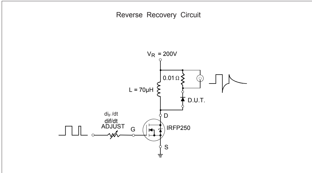
Fig. 9- Reverse Recovery Parameter Test Circuit
