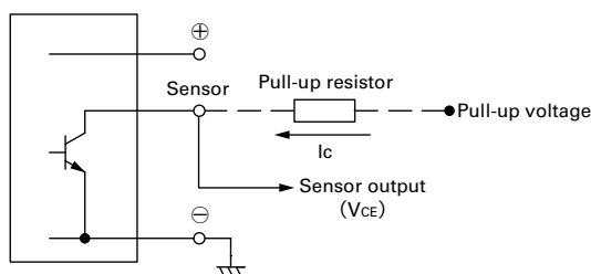
Inside of DC fan
