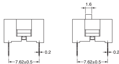
Flat Actuator
