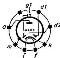
Sockelschaltenschema
