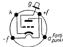
Schaltschema
