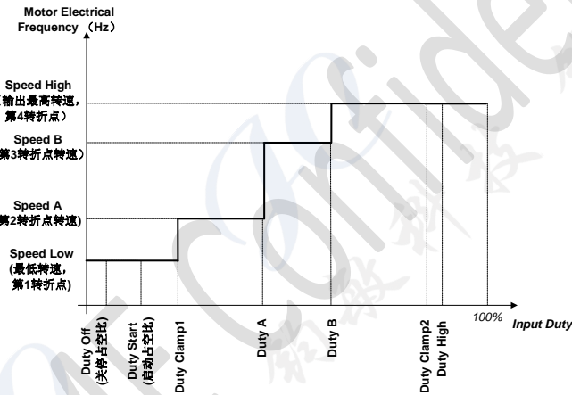
图 15 小占空比不断断模式 (Register 0x26 [4]=1, Register 0x27 [2]=1)
